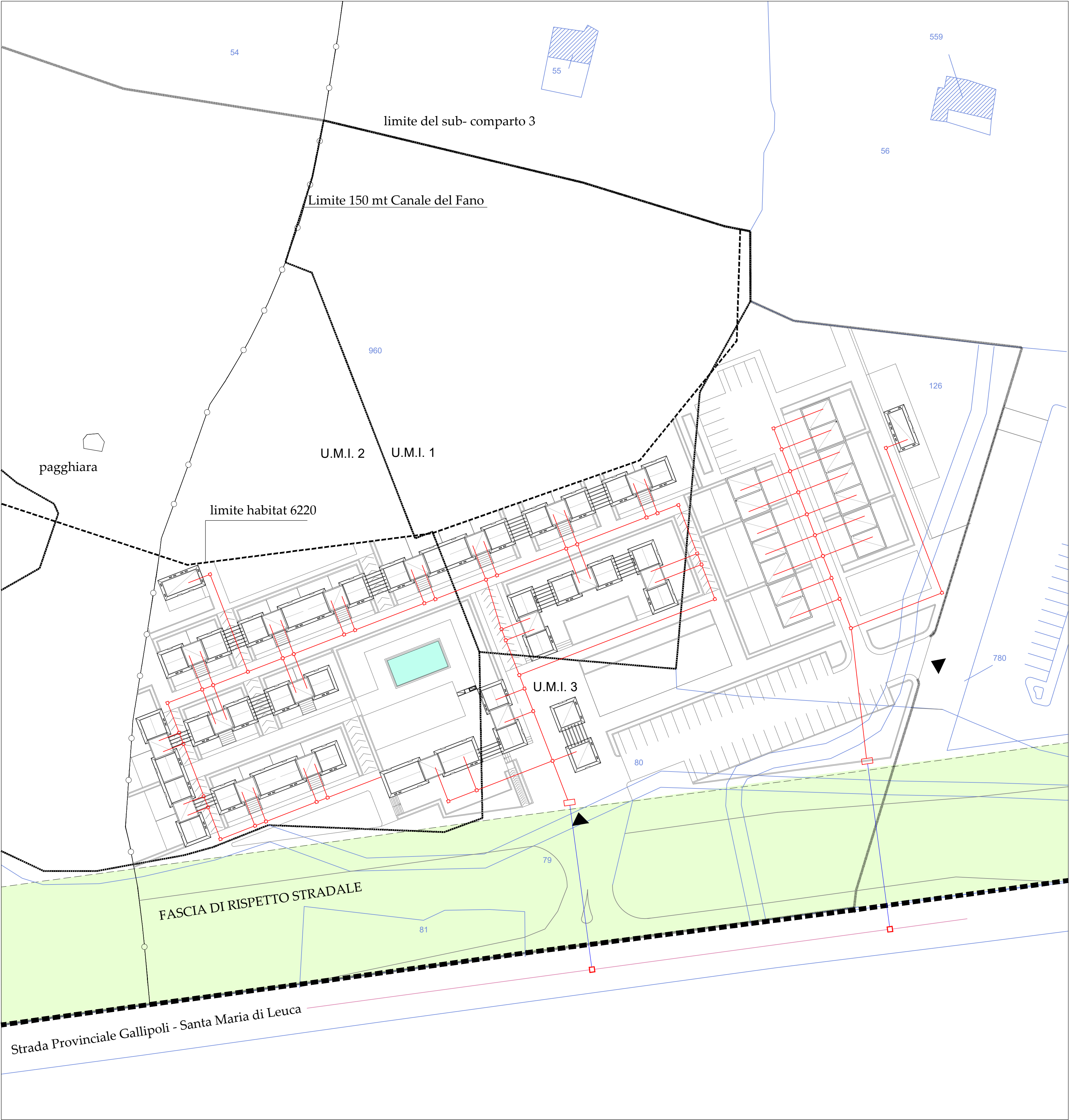
PLANIMETRIA GENERALE RETE IDRICA - scala 1: 500
